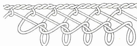
Skematisk tegning af guldtrådsbroderi. Øverst nr. 65, nederst nr. 449. (Tegninger: K. Thorvildsen 1957, s. 80)
