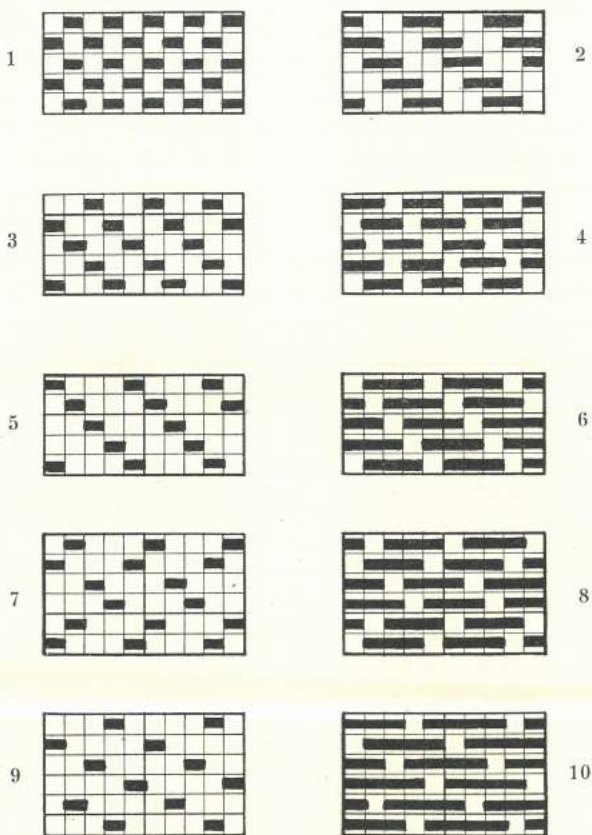
Fig. 1. 1. Toskaft. 2. Firskaftet Dobbeltkipper. 3, 5 7 og 9 er Bolsterbindinger (Trendeffekt). 4, 6, 8 og 10 er Olmerdugsbindinger (Skudeffekt).
